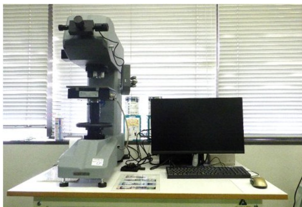
ビッカース硬さ試験機
