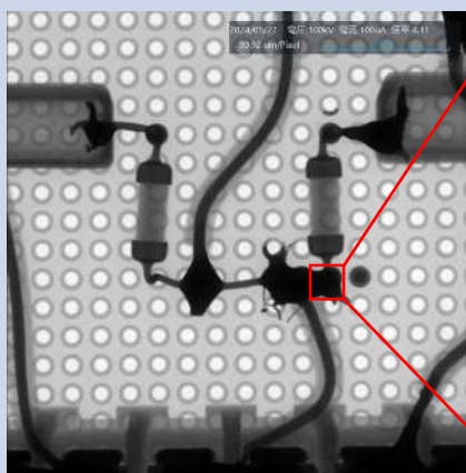
電子基板(X線透過画像)
